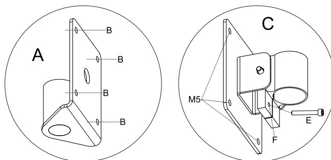
VERVE 108A / 108
